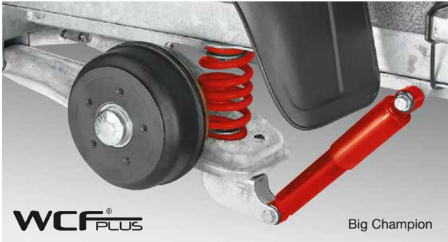
Rijcomfort dankzij het World-Class-chassis volgens automobielstandaard met wielschokbrekers en Tempo 100-ontheffing (geldt voor Duitsland).
